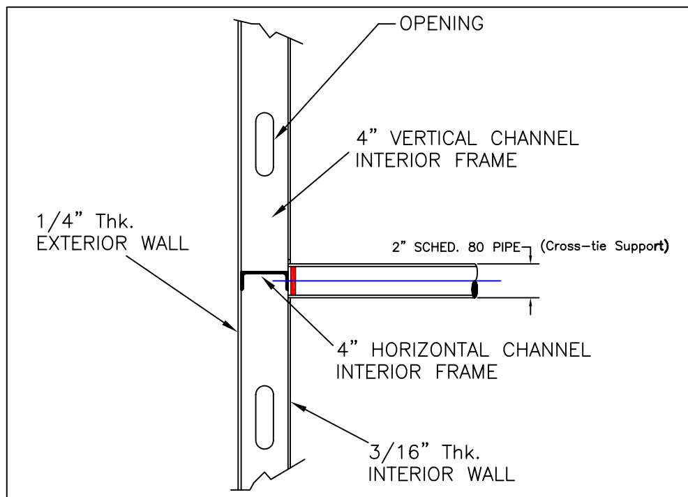
VIEW A-A
